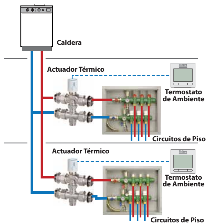
b) Con Válvula de 3 vías con Bypass fuera del gabinete
